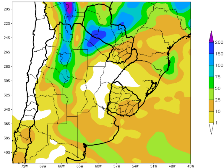
PERSPECTIVA DEL 15 AL 21 DE DICIEMBRE DE 2022 PRECIPITACION (mm)
