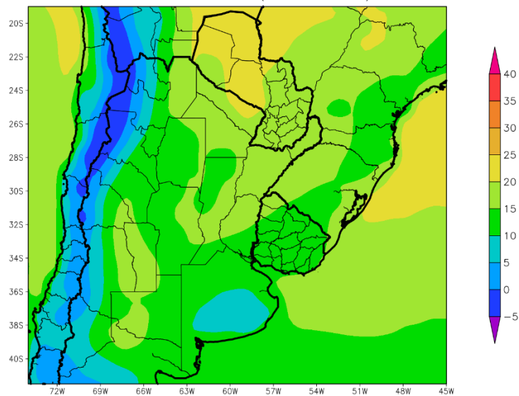
PERSPECTIVA DEL 15 AL 21 DE DICIEMBRE DE 2022 TEMPERATURA MINIMA(Grados Cent.)
