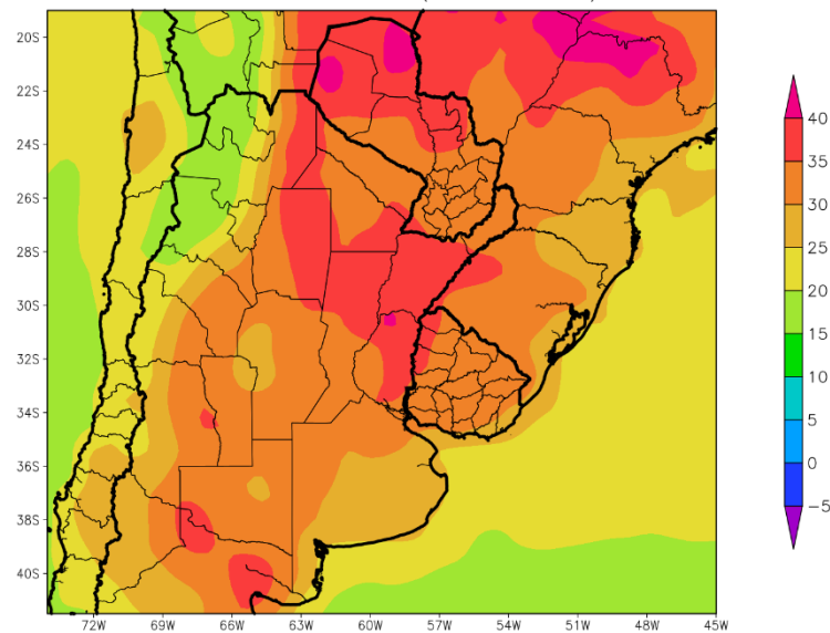
PERSPECTIVA DEL 15 AL 21 DE DICIEMBRE DE 2022 TEMPERATURA MAXIMA(Grados Cent.)
