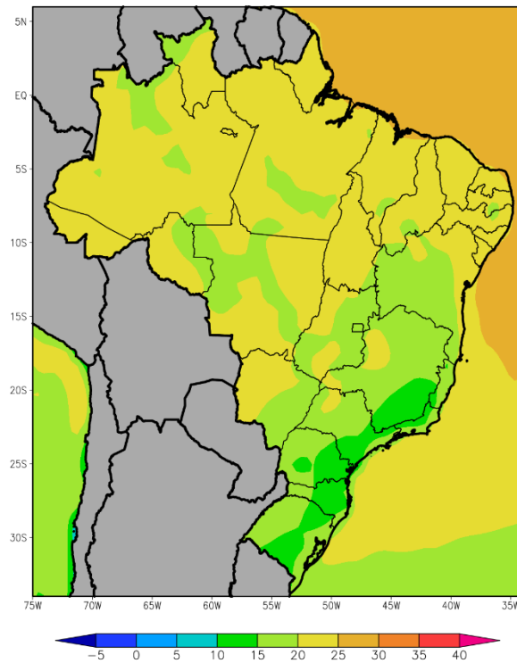
PERSPECTIVA DEL 15 AL 21 DE DICIEMBRE DE 2022 TEMPERATURA MINIMA(Grados Cent.)
