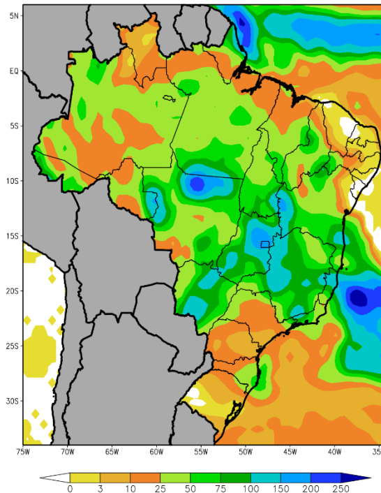
PERSPECTIVA DEL 15 AL 21 DE DICIEMBRE DE 2022 PRECIPITACION (mm)
